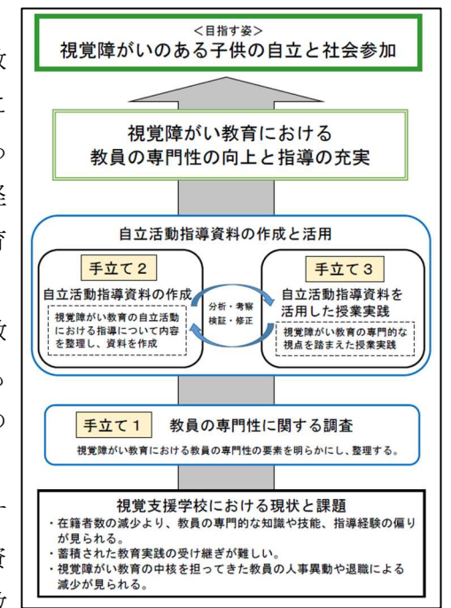
【研究構想図】
