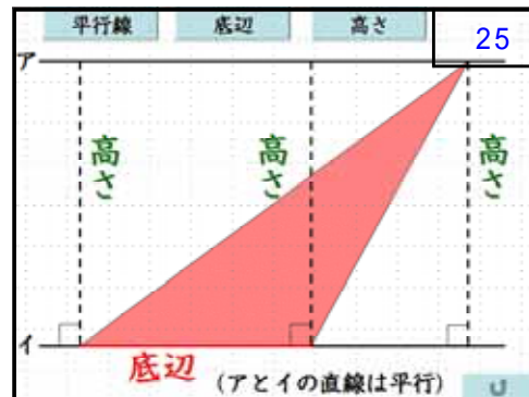
【図78】底辺と高さの関係
